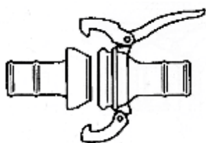
TACHYSYNDΕΣΜΟΣ ΜΑΝΙΚΑΣ
